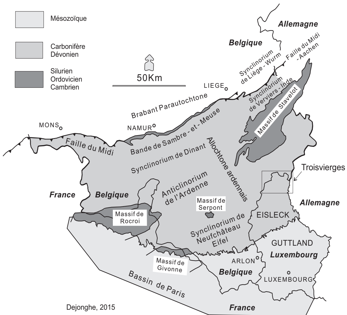
Figure 2 : Localisation de la carte de Troisvierges et des principales unités structurales concernées.
