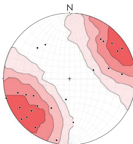
Figure 8 : Stéréogramme des axes des pôles des plans de diaclases (ronds, N = 26 ), angles conservés.
